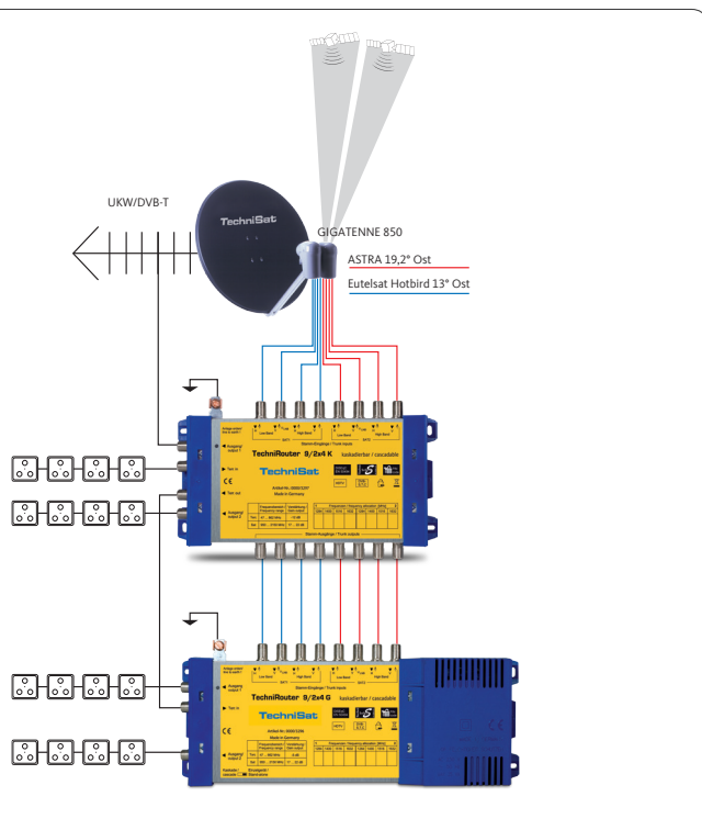
Installationsbeispiel
