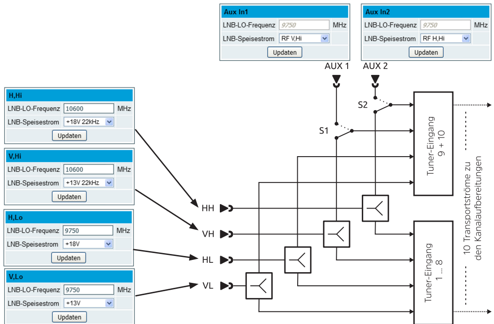
Abb. 8.3-1: LNB-Einstellungen, Beispiel mit Quattro-Switch-LNB, AUX-Eingänge nicht genutzt.
