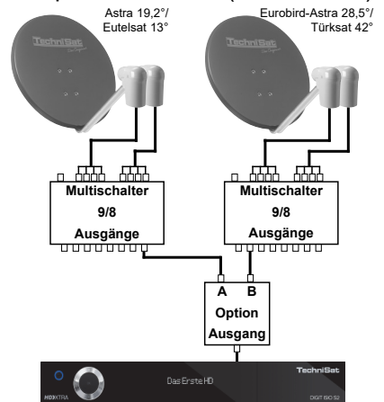
Beispiel 3: 4 Satelliten (Quattro-LNBs)
