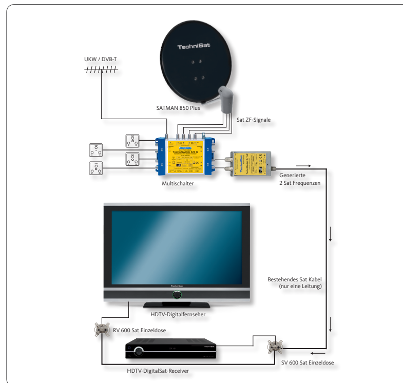
Installationsbeispiel für 2 Einzelteilnehmer
