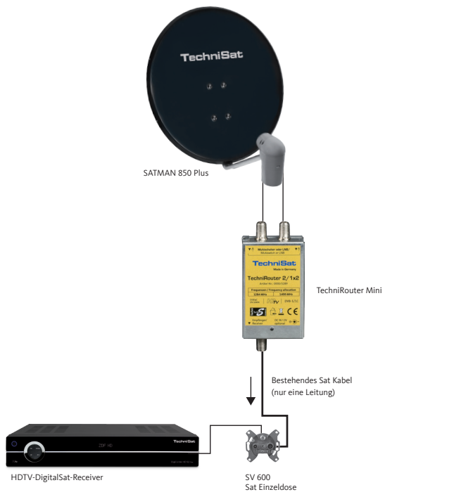
Installationsbeispiel für 1 Anschluss an einen Twin-Receiver
