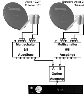
Beispiel 3: 4 Satelliten (Quattro-LNBs) Astra 19,2° Eutelsat 13° Eurobird-Astra 28,5° Türksat 42°
